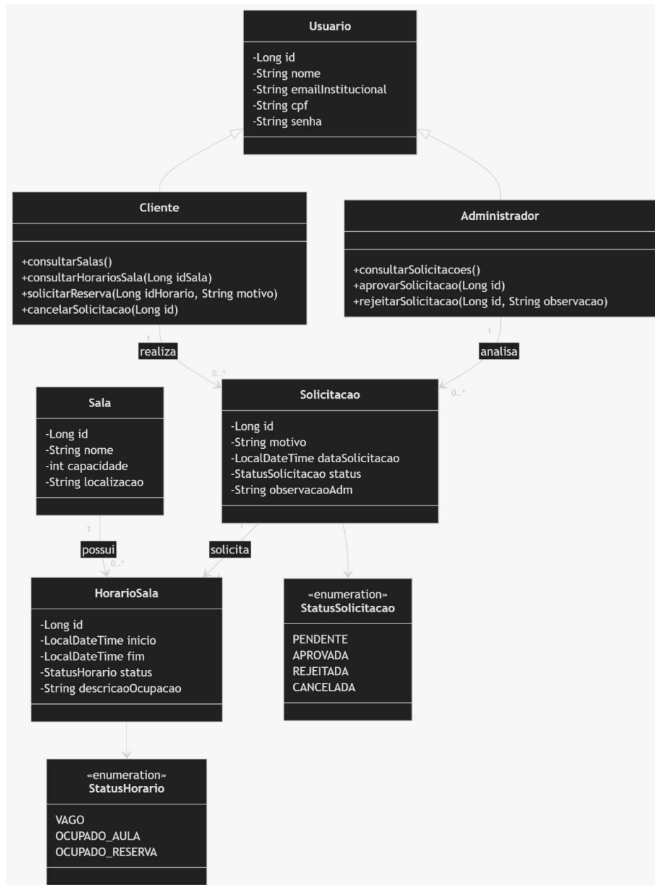
Figura 5 - Diagrama de Classes
